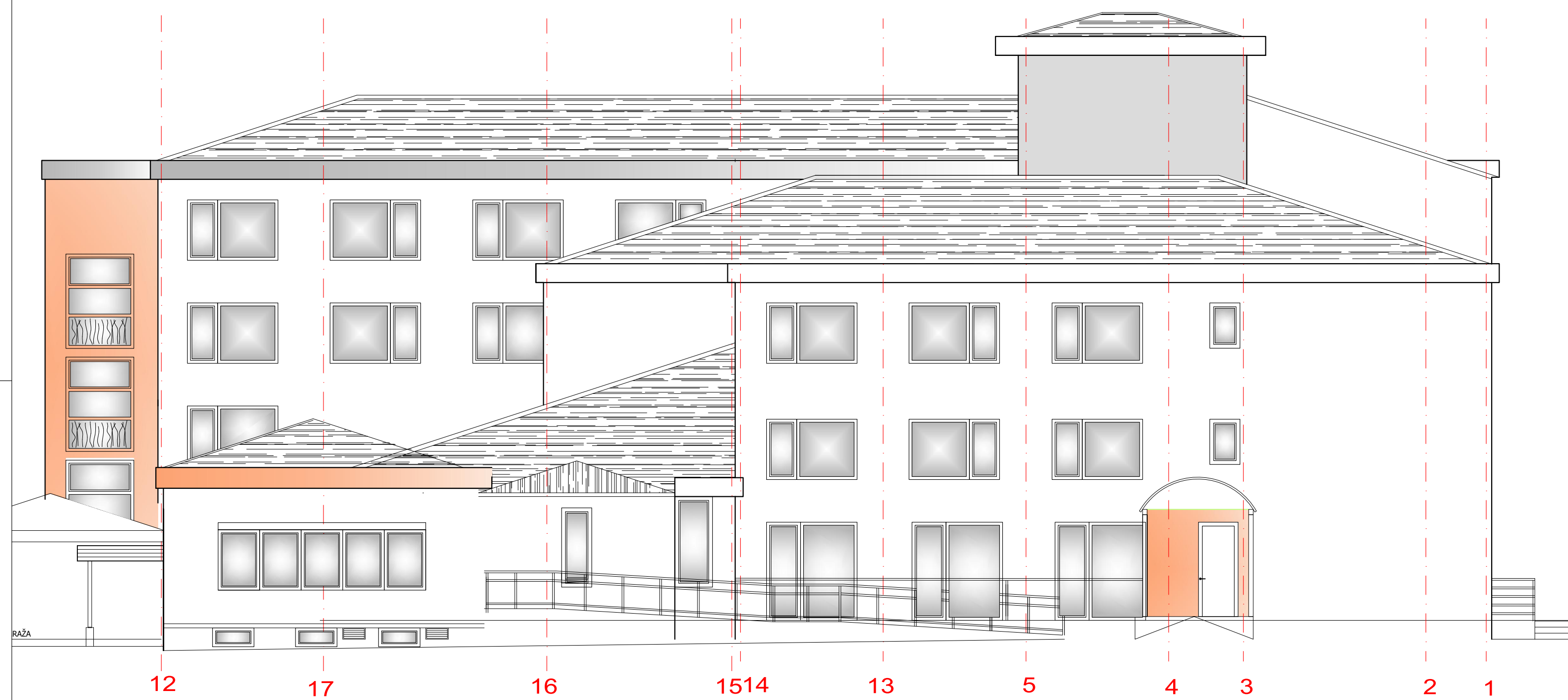
FASADA ZAHOD
