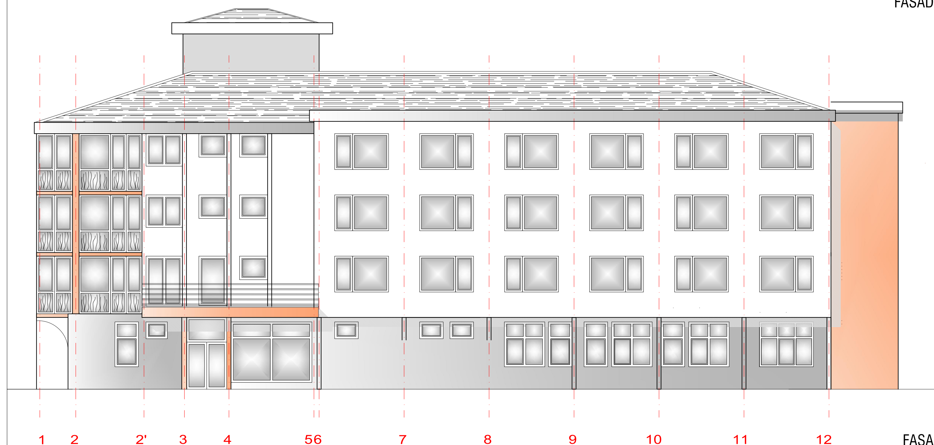
FASADA ZAHOD
